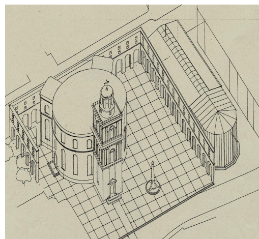
Abb. 129: Frankfurt. Paulsplatz. Wettbewerb 1983. Entwurf Goldapp und Klumpp.
