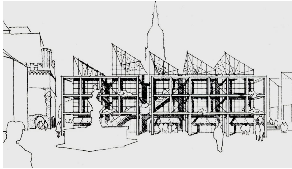
Abb. 113: Frankfurt. Römerberg. Wettbewerb 1980. Alternativentwurf von Gerkan, Marg + Partner ohne „Historische Ostzeile“.
