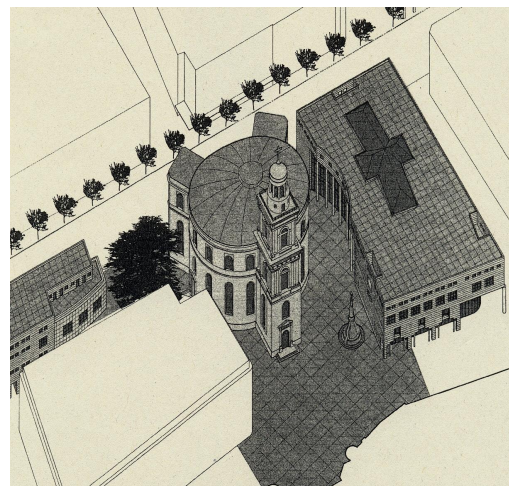
Abb. 127: Frankfurt, Paulsplatz. Wettbewerb 1983. Entwurf Bartsch, Thürwächter, Weber.
