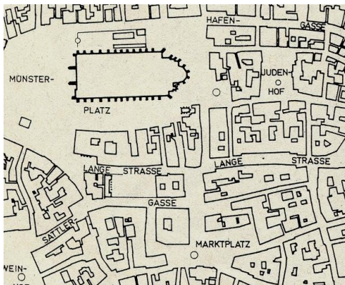
Abb. 480: Ulm. Stadtkern mit Münsterplatz und Marktplatz nach dem Abriß des Barfüßerklosters (Zustand 1926).
