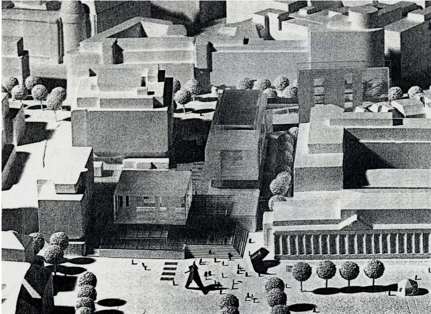
Abb. 462: Stuttgart. Schloßplatz / Kleiner Schloßplatz. Wettbewerb 1998 / 1999. Entwurf Hascher / Jehle.
