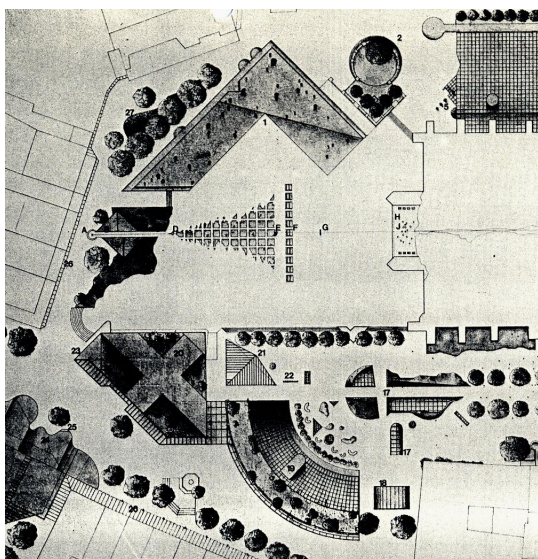
Abb. 495: Ulm. Münsterplatz. Projekt „Ulm neu“, Schaal / Hess 1975. Lageplan (Ausschnitt); das Münster am rechten Bildrand.
