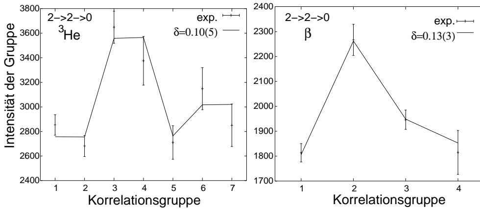
Abbildung 4.2: Bestimmung des Multipolmischungsverhältnisses \delta(2_3^+ \rightarrow 2_1^+) im ^3\text{He} -Experiment (links) und im \beta -Zerfallsexperiment (rechts) über Auswertung der Winkelkorrelation. Die Gruppen sind in Abschnitt 3.3.4 auf Seite 29 beschrieben, die Zählraten in den Gruppen stammen aus den über die Ansprechwahrscheinlichkeit korrigierten Zählraten des Schnitts auf den 833 keV Übergang in Koinkidenz zum 1451 keV Übergang.
