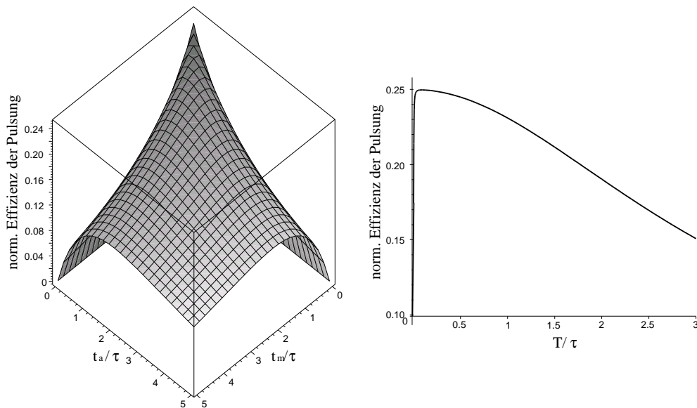
Abbildung 3.7: Darstellung der Effizienz der Pulsung. Auf dem linken Bild erkennt man, dass gleichlange Mess- ( t_m ) und Anregungszeiten ( t_a ) die Effizienz der Pulsung erhöhen. Auf der rechten Grafik sieht man die Abhängigkeit der Effizienz von der Zyklusdauer von T = t_m + t_a + \text{Schaltzeit} mit t_m = t_a . Die Schaltzeit ist hierbei eine feste 5 ms lange elektronische Konstante. Ein flaches Maximum bei Schaltzeiten mit T < \tau und T > \text{Schaltzeit} ist zu erkennen. Normiert wurde jeweils auf die bei durchgehendem Strahlbetrieb und gleichem Strom angeregten Kerne.
