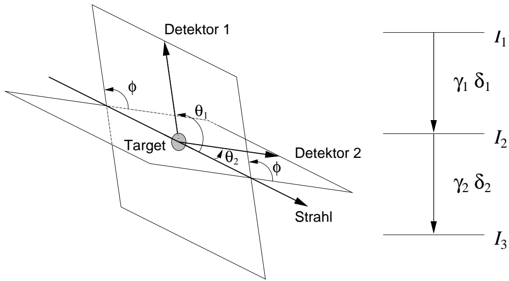
Abbildung 3.14: Beschreibung der Winkel der Detektoren bei der Winkelkorrelation. Rechts sind zusätzlich die Bezeichnungen einer \gamma\gamma -Koinzidenz angegeben.
