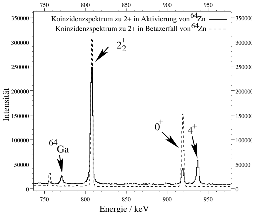
Abbildung 3.6: Vergleich zwischen der Messung bei Anregung des Kerns ^{64}\text{Zn} und bei \beta -Zerfall zu ^{64}\text{Zn} . Deutlich zu erkennen ist die schmalere Halbwertsbreite der Peaks und somit die bessere Energieauflösung sowie das Fehlen von Kontaminationen, wie es im Fall der Anregungsmatrix bei ^{64}\text{Ga} der Fall ist. Zudem erkennt man, dass nicht alle Niveaus durch den \beta -Zerfall bevölkert werden. Aufgrund der Auswahlregeln werden nur 0^+ und 1^+ Zustände direkt bevölkert. Tiefliegende Zustände höherer Spins werden indirekt bevölkert. Nicht bevölkert werden Zustände mit J > 1 bei hohen Energien, wie z.B. der 4_2^+ mit dem Zerfall über die 937 keV Linie.
