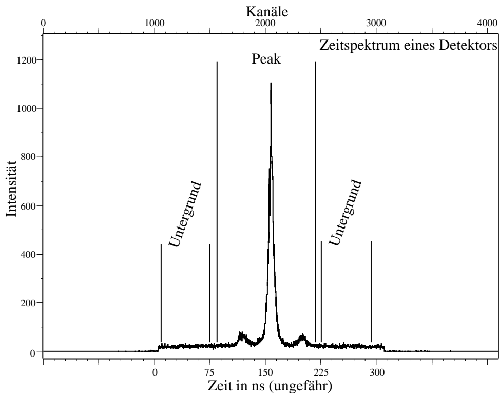
Abbildung 3.12: Zeitspektrum eines Detektors in Relation zu einem zweiten Detektor. Etwa 150 ns nachdem der zweite Detektor das Zeitfenster geöffnet hat, registriert der erste Detektor ein Signal. Über das Peakfenster und die Untergrundfenster können zufällige Koinzidenzen eliminiert werden. Die Breiten der beiden Untergrundfenster müssen dazu insgesamt die Breite des Peakfensters haben.
