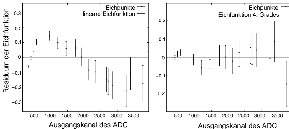
Abbildung 3.10: Abweichungen der Eichfunktion von den gemessenen Eichlinien der ^{226}\text{Ra} Quelle. Es werden hier exemplarisch die Eichfunktion und die Eichpunkte des Mittelsegments des CLUSTERS bei der ( ^3\text{He} , 2n)-Messung betrachtet. Im linken Bild erkennt man starke Abweichungen der Eichlinien von der linearen Eichfunktion. Im rechten Bild wurde deshalb eine Eichfunktion vierten Grades gewählt. Somit liegt der Fehler der Energieeichung bei unter 0.01%.
