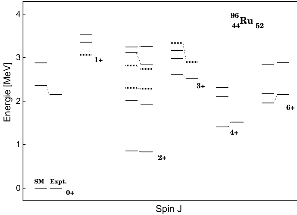
Abbildung 4.7: Vergleich des berechneten und gemessenen Termschemas der J^+ = 0^+ \dots 6^+ Zustände in ^{96}\text{Ru} . Zustände gemischter Symmetrie sind gestrichelt eingezeichnet.
