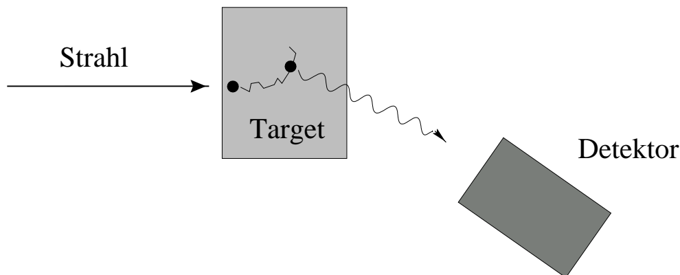
Abbildung 3.16: Darstellung des Messaufbaus zur DSAM-Methode. Der Projektilstrahl trifft das Target und bildet einen Compound-Kern, der nach Abdampfung einiger Neutronen im Target abgebremst wird. Während der Abbremsung werden \gamma -Quanten abgestrahlt, die von den Detektoren aufgezeichnet werden.
