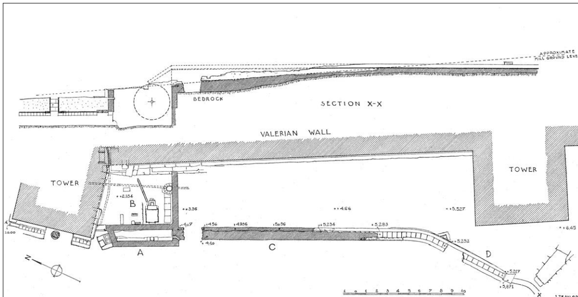
1 Agora greca, il mulino centrale, planimetria
