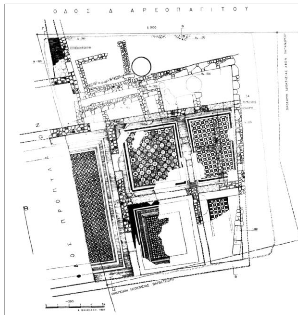
1 Abitazione scoperta all'incrocio tra O. Dionisiou Areopagitou e O. Propylaiōn
