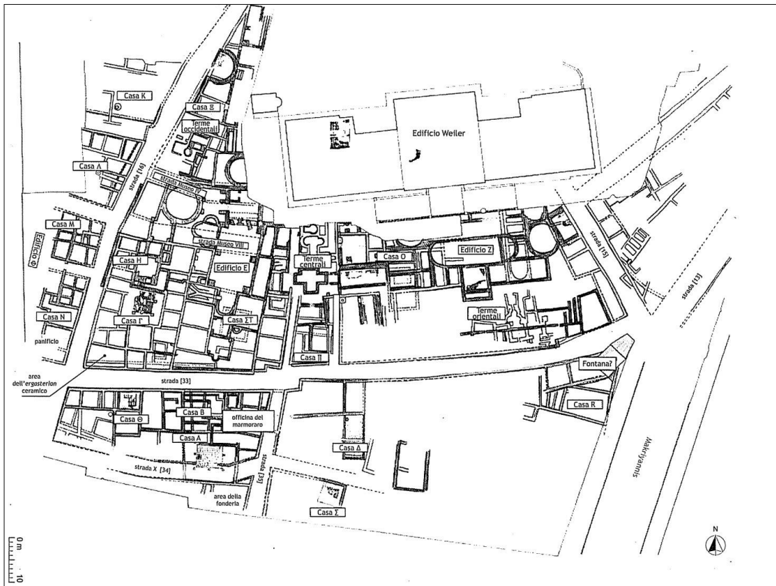
1 Quartiere a sud dell'Acropoli, area di scavo sotto il nuovo Museo dell'Acropoli
