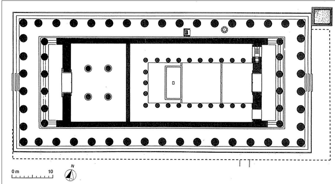
1 Partenone, planimetria ricostruttiva
