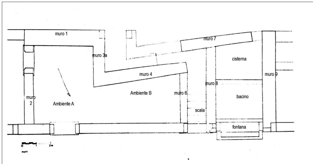
1 Agora romana, portico interno meridionale. Complesso di vani con fontana nella fase originaria
