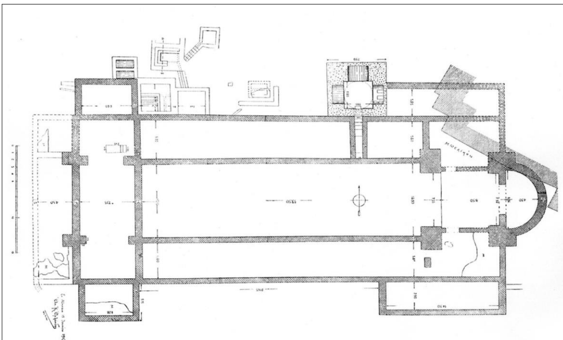
1 Basilica dell'Ilisso con annesso martyrion
