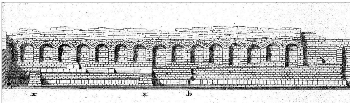
2 La Stoa di Eumene, il muro ad arcate e il muro di fondo della stoa con addossati due pilastri attribuiti all'età tardo antica (X)
