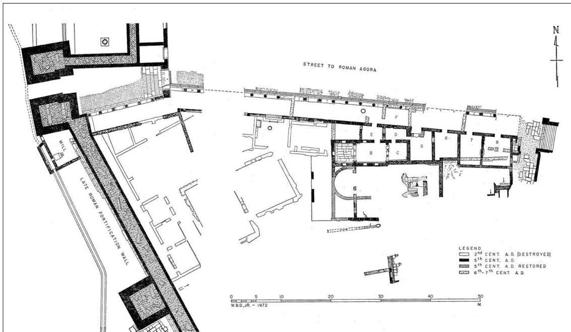
1 Edificio ad est della Biblioteca di Pantainos, planimetria
