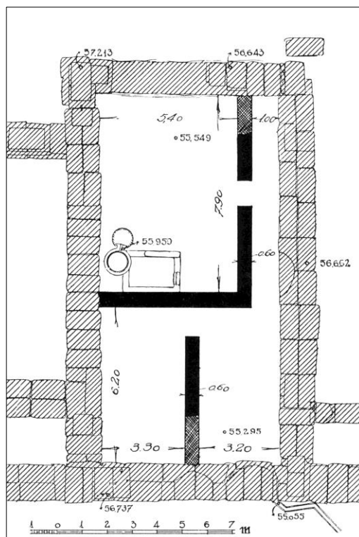
2 Il terzo vano da sud nel Mētrōon in seguito alla costruzione della pressa per l'olio, planimetria
