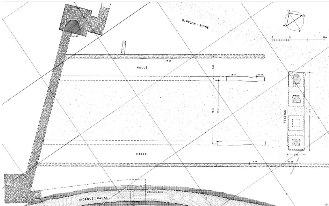
1 Le fondazioni della Hallenstraße e Festtor
