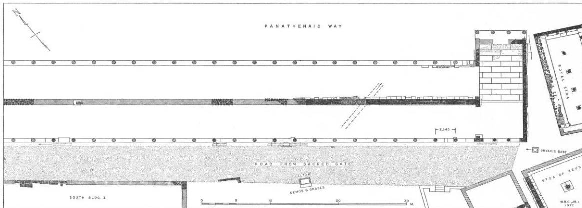
1 Stoa sul lato meridionale della Via Panatenaica, ricostruzione planimetrica della struttura del I-III sec. d.C.
