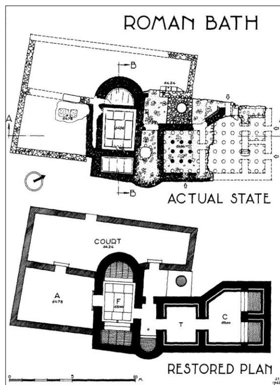
1 Areopago, Terme orientali, planimetria generale dei resti e planimetria ricostruttiva
