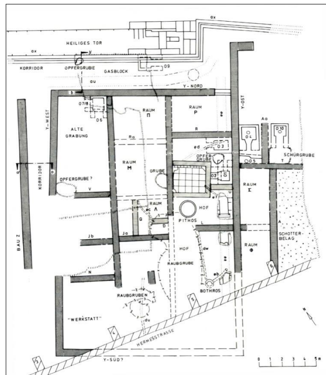
1 Il Bau Y, planimetria successiva al ripristino del V sec. d.C.
