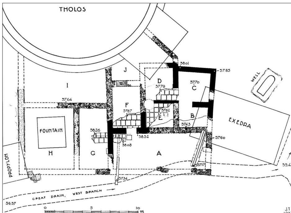
2 La casa addossata alla Tholos, planimetria
