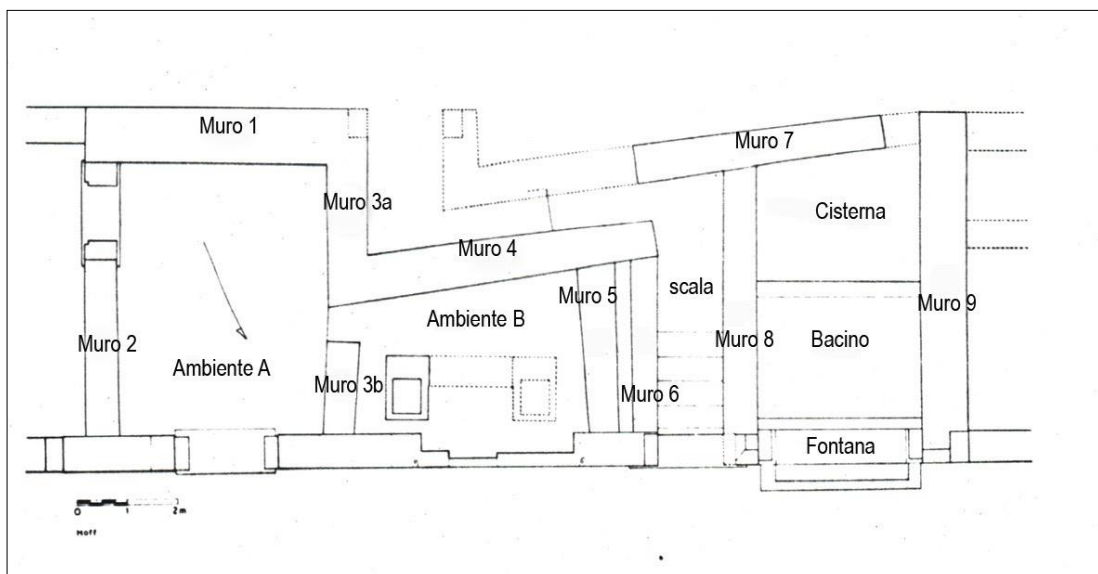
2 Agora romana, portico interno meridionale. Complesso di vani con fontana in seguito agli interventi attribuibili all'età tardo antica
