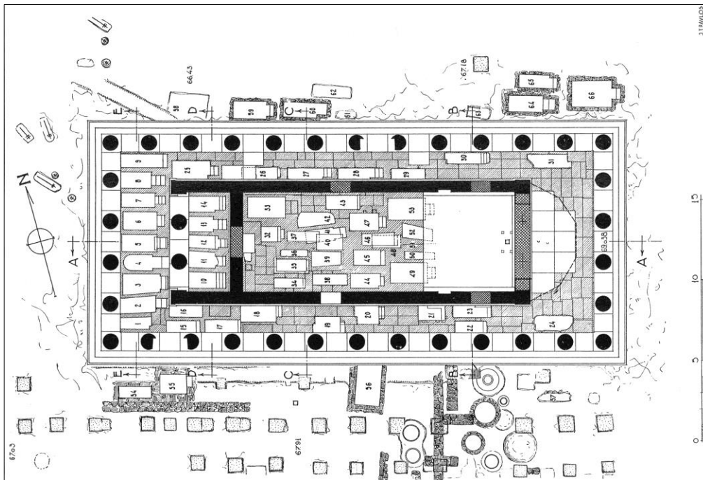
1 Agora greca, Tempio di Efesto in seguito alla conversione in chiesa, planimetria
