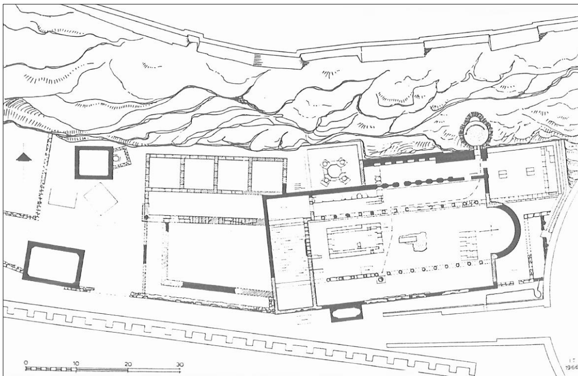
2 La basilica tardo antica costruita all'interno del santuario di Asclepio alle pendici meridionali dell'Acropoli, planimetria ricostruttiva (Traulos 1939-1941, 39 fig. 4)
