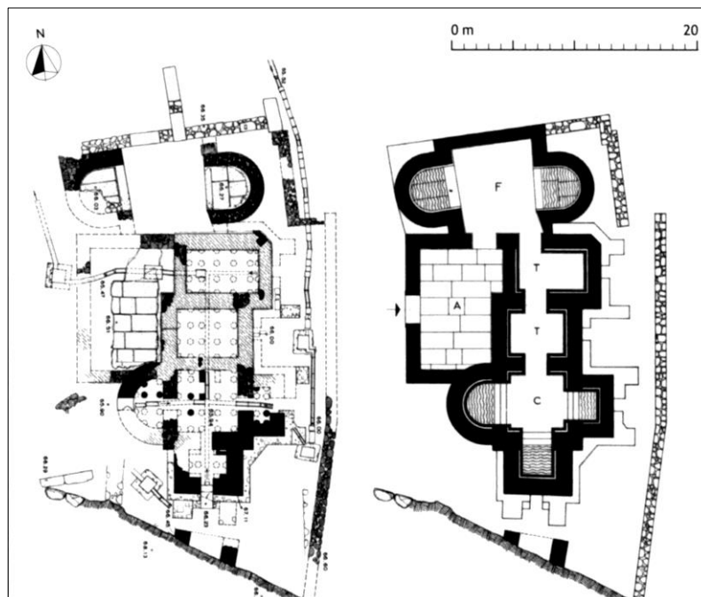
2 Areopago, la Terme settentrionali, planimetria dei resti e planimetria ricostruttiva
