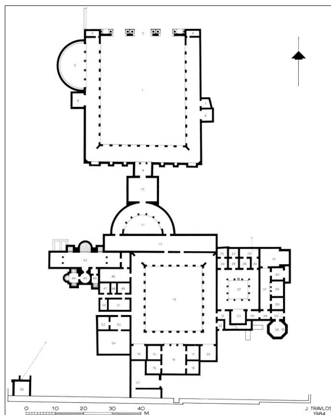
1 Agora greca, Palazzo dei Giganti, planimetria ricostruttiva
