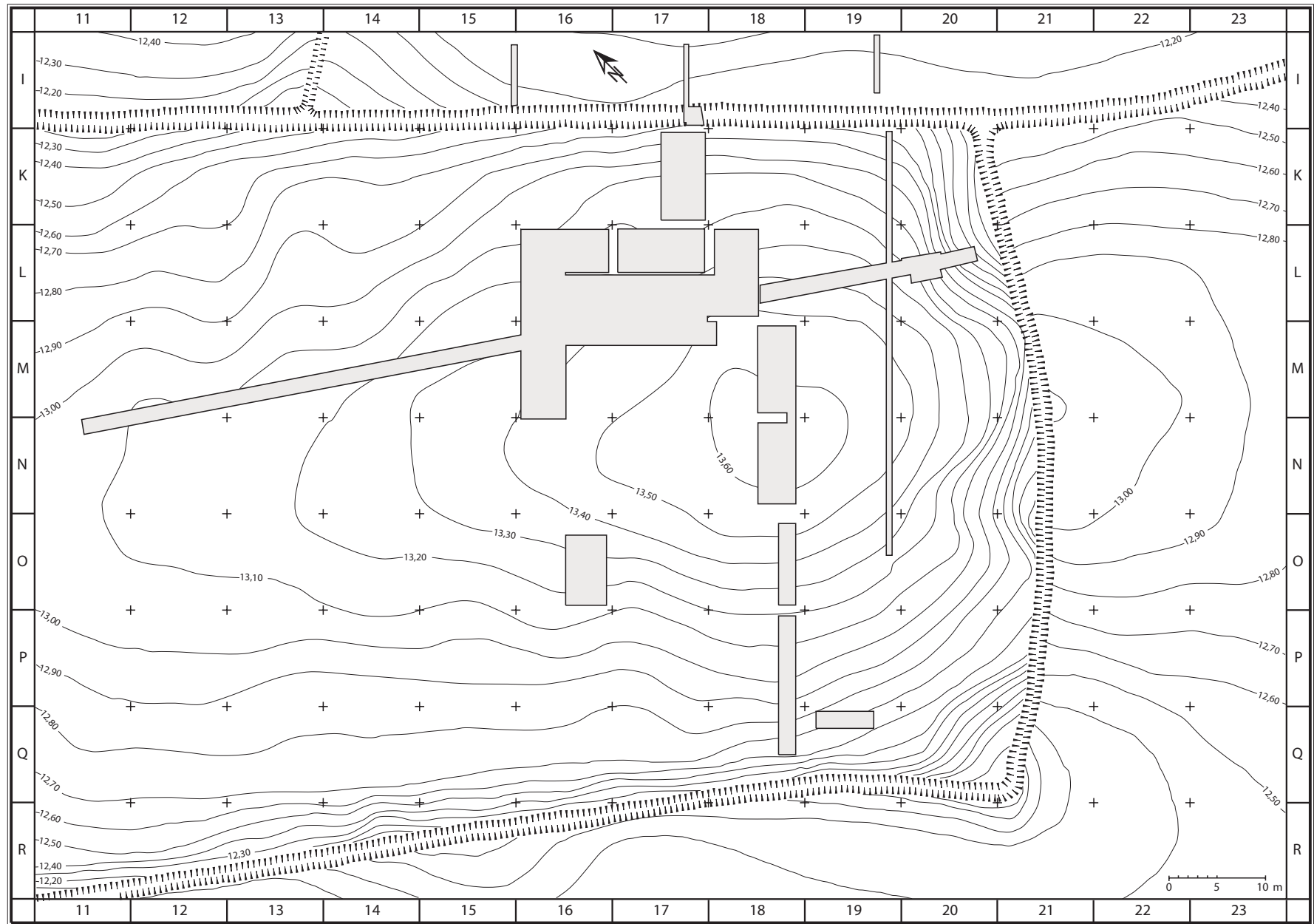
Abb. 2 Este-Santuario di Reitia. Fondo Baratella (Schnitt- und Flächenplan).
