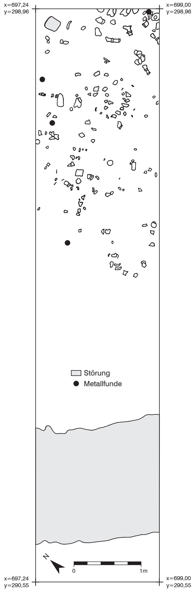
Abb. 37 Este-Santuario di Reitia. Gesamtplan der Fläche O18 mit Keramik aus den Perioden Este III Mitte bis Anfang Este III Spät.
