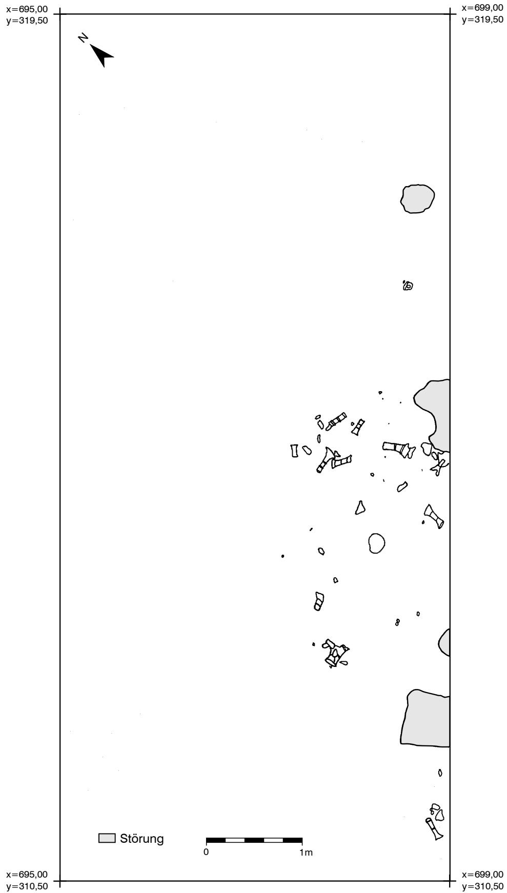
Abb. 35 Este-Santuario di Reitia. Gesamtplan der Fläche M18 mit Keramik aus der Periode Este III Früh.
