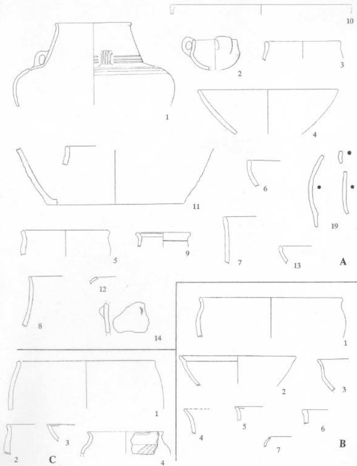
A: St. 8007, B: St. 8046, C: St. 8017 (alle M 1:4).
