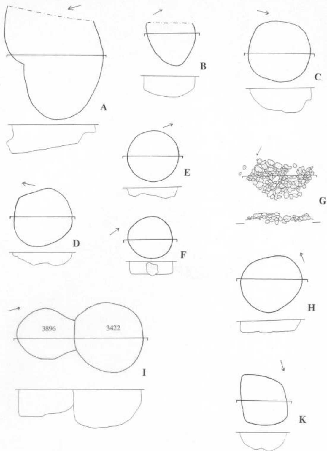
A: St. 3330, B: St. 3336, C: St. 3409, D: St. 3410, E: St. 3412, F: St. 3413, G: St. 3444, H: St. 3470, I: St. 3422 und 3896, K: St. 3484 (alle M 1:50).
