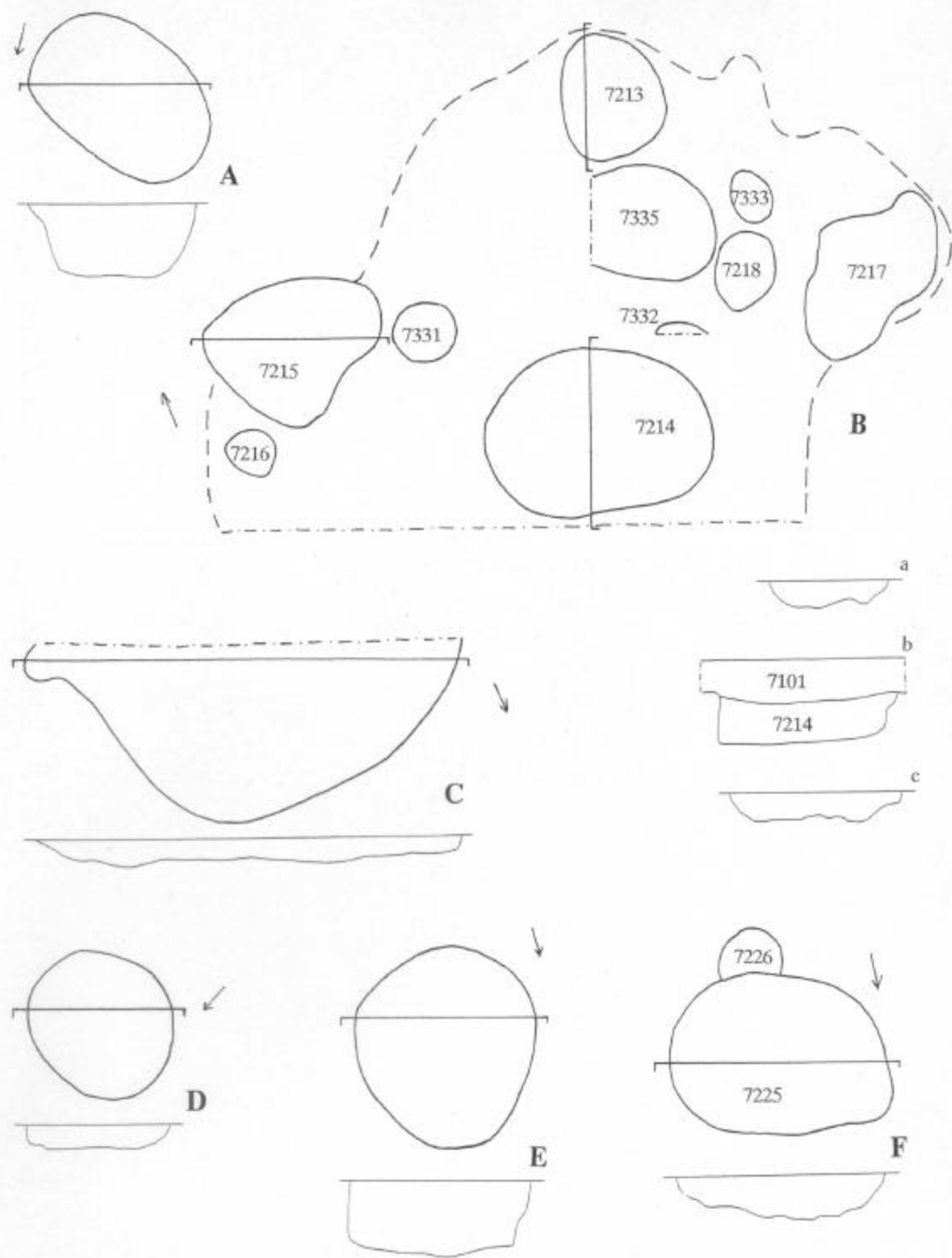
A: St. 7018, B: Grubenkomplex St. 7101, a: Profil St. 7213, b: Profil St. 7101 und 7214, c: Profil St. 7215, B: St. 7110, C: St. 7107, D: St. 7160, E: St. 7225 und 7226 (alle M 1:50).
