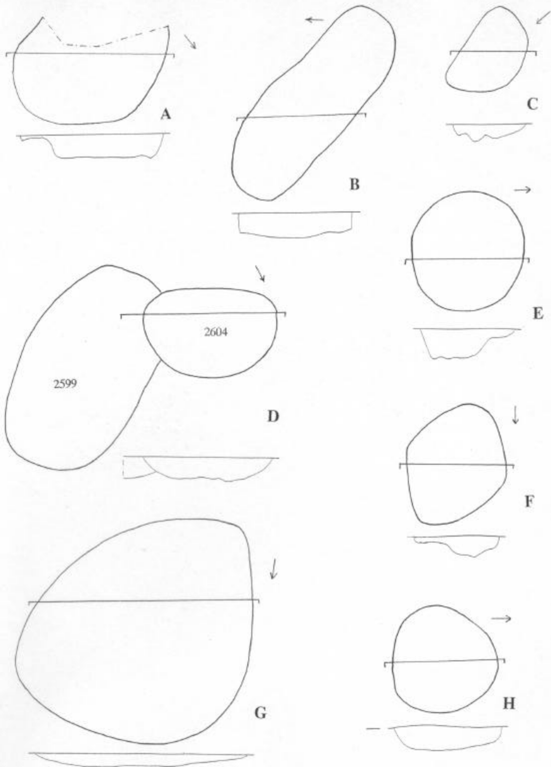
A: St. 2594, B: St. 2595, C: St. 2626, D: St. 2599 und 2604, E: St. 2621, F: St. 2627, G: St. 2636, H: St. 2696 (alle M 1:50).
