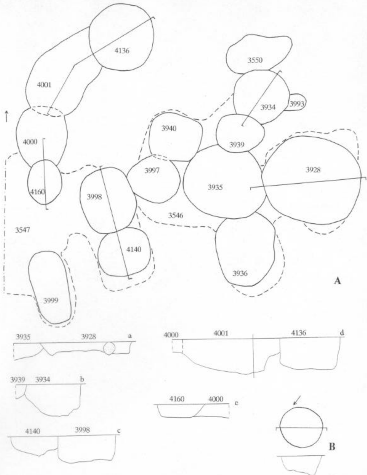
A: Grubenkomplexe St. 3546 und 3547, a: Profil St. 3928 und 3935, b: Profil St. 3934 und 3939, c: Profil St. 3998 und 4140, d: Profil St. 4000, 4001 und 4136, e: Profil St. 4000 und 4160, B: St. 3572 (alle M 1:50).
