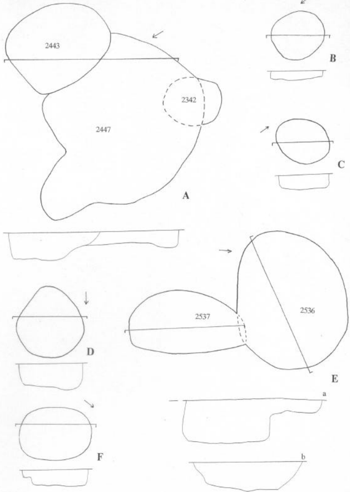
A: St. 2342, 2443 und 2447, B: St. 2554, C: St. 2557, D: St. 2570, E: St. 2536 und 2537, a: Profil St. 2536, b: Profil St. 2537, F: St. 2596 (alle M 1:50).
